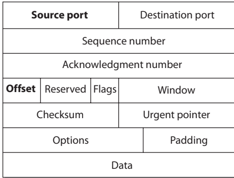
TCP format
