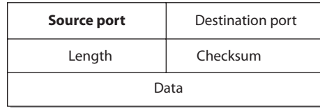
UDP format
